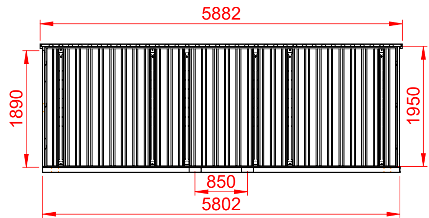
B-B SCALE 1 : 60
