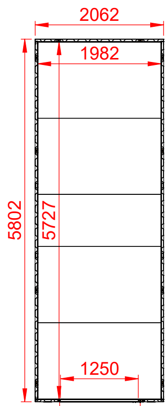
A-A SCALE 1 : 60
